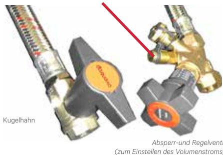
Entleerungs- und Entlüftungsventil sowie Messanschluss (für die Messung des Wasserdurchflusses)
